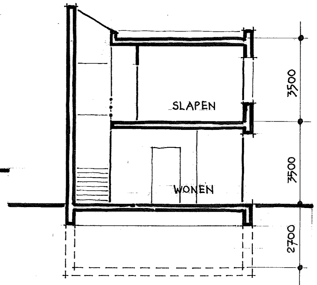
DWARSDOORSNEDE
