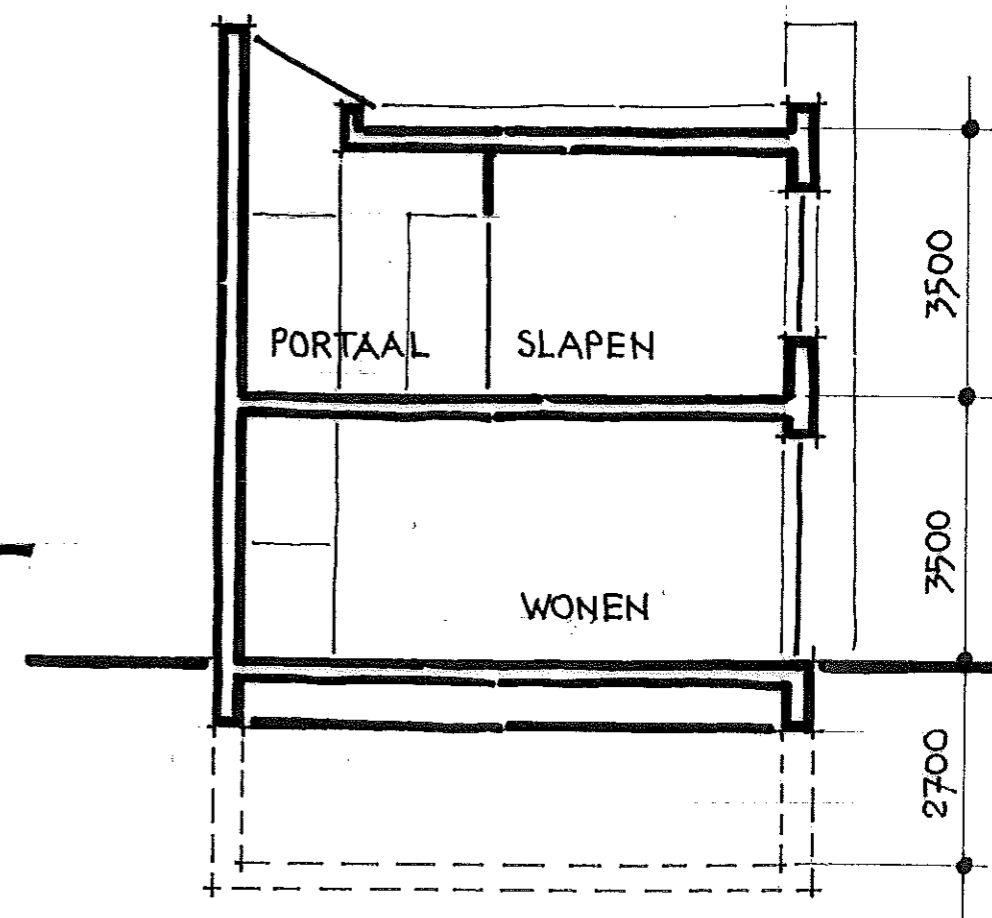
DWARSDOORSNEDE
