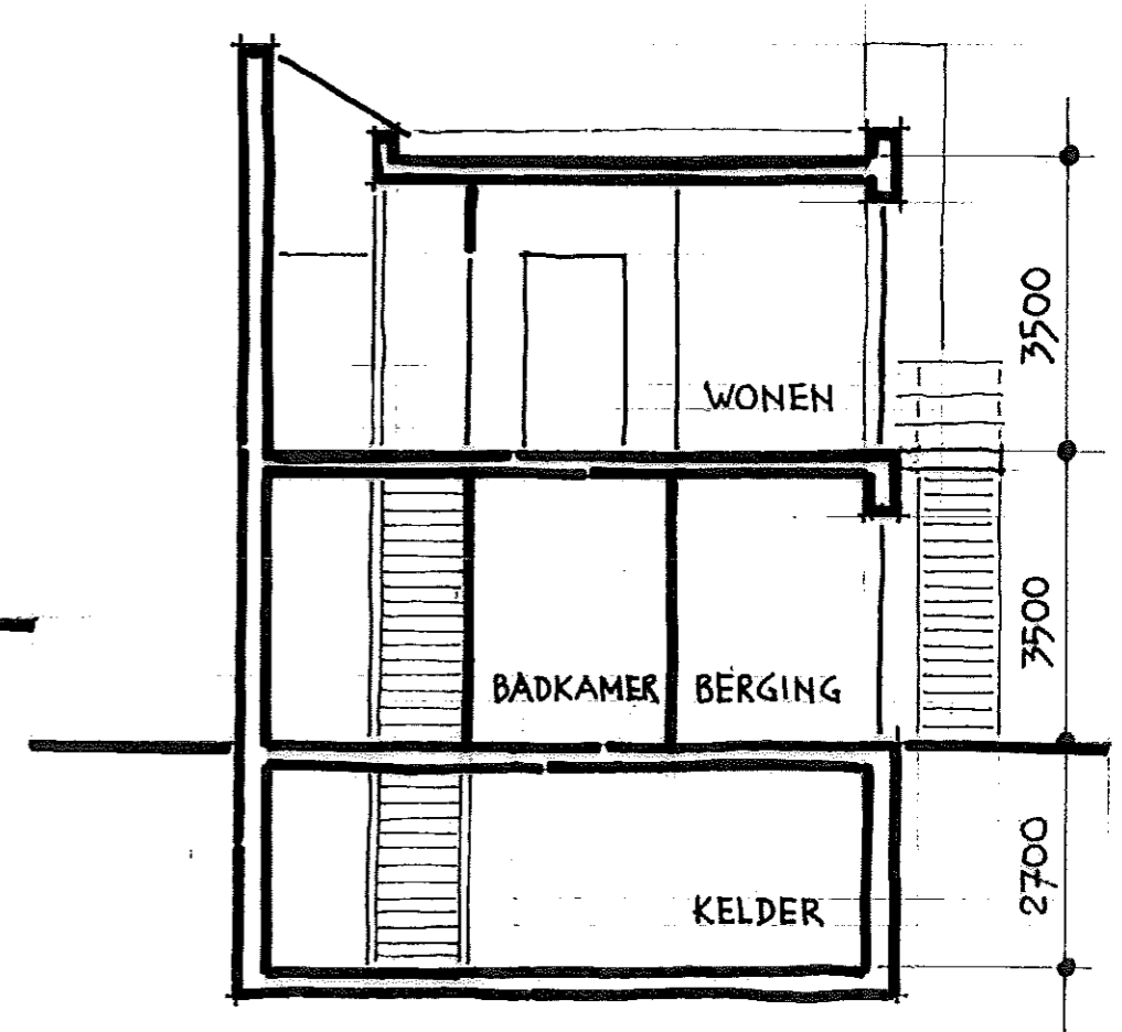
DWARSDOORSNEDE
