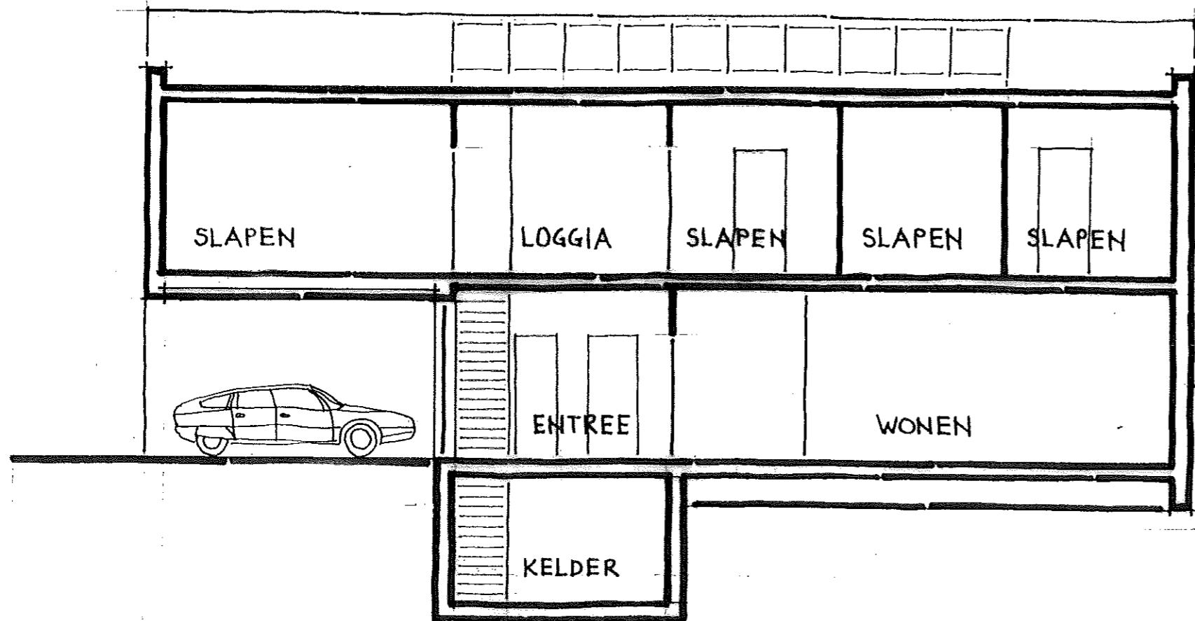
LANGSDOORSNEDE
