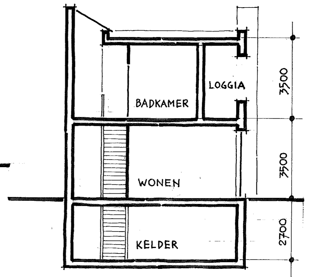
DWARSDOORSNEDE
