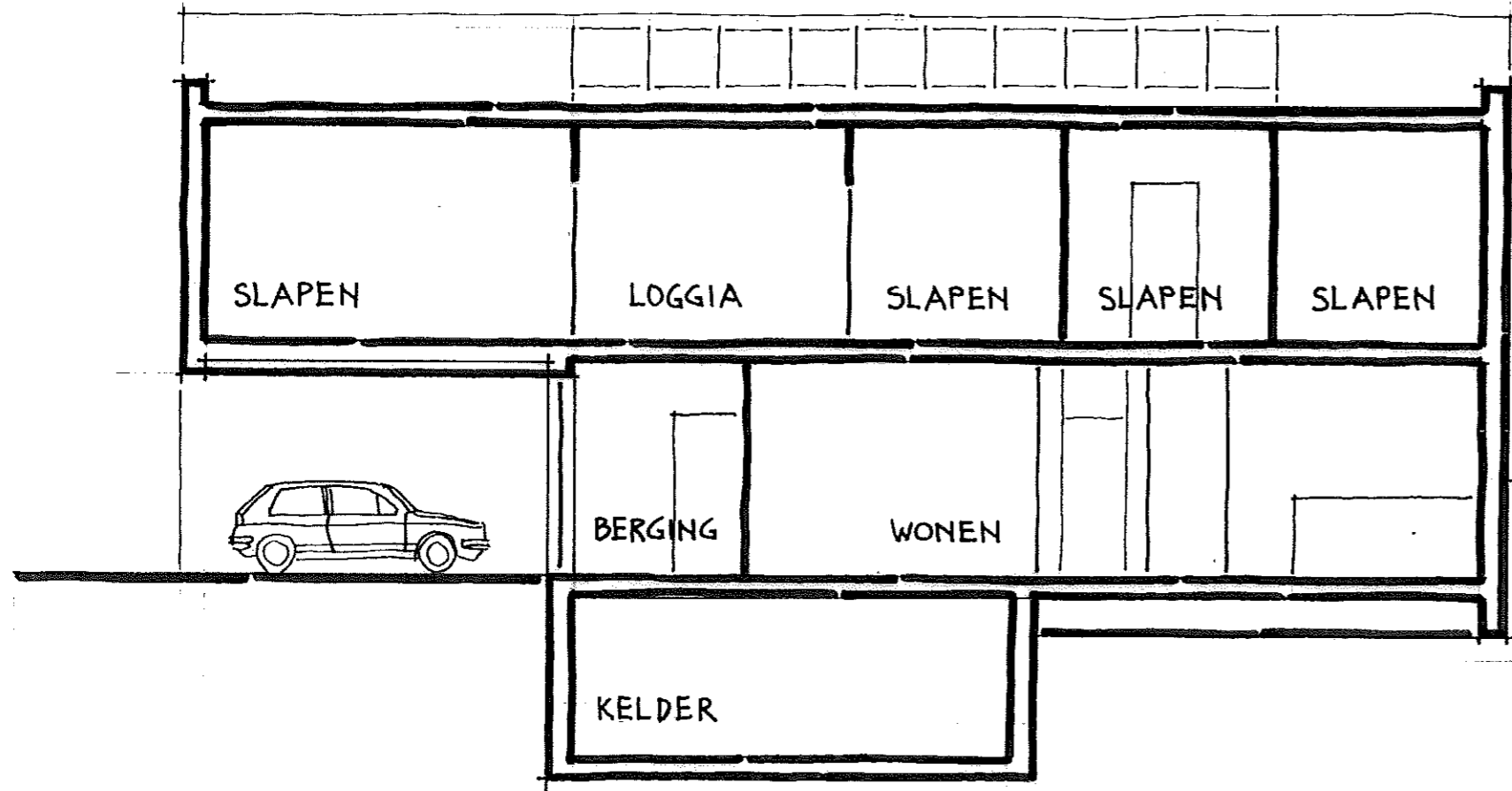
LANGSDOORSNEDE
