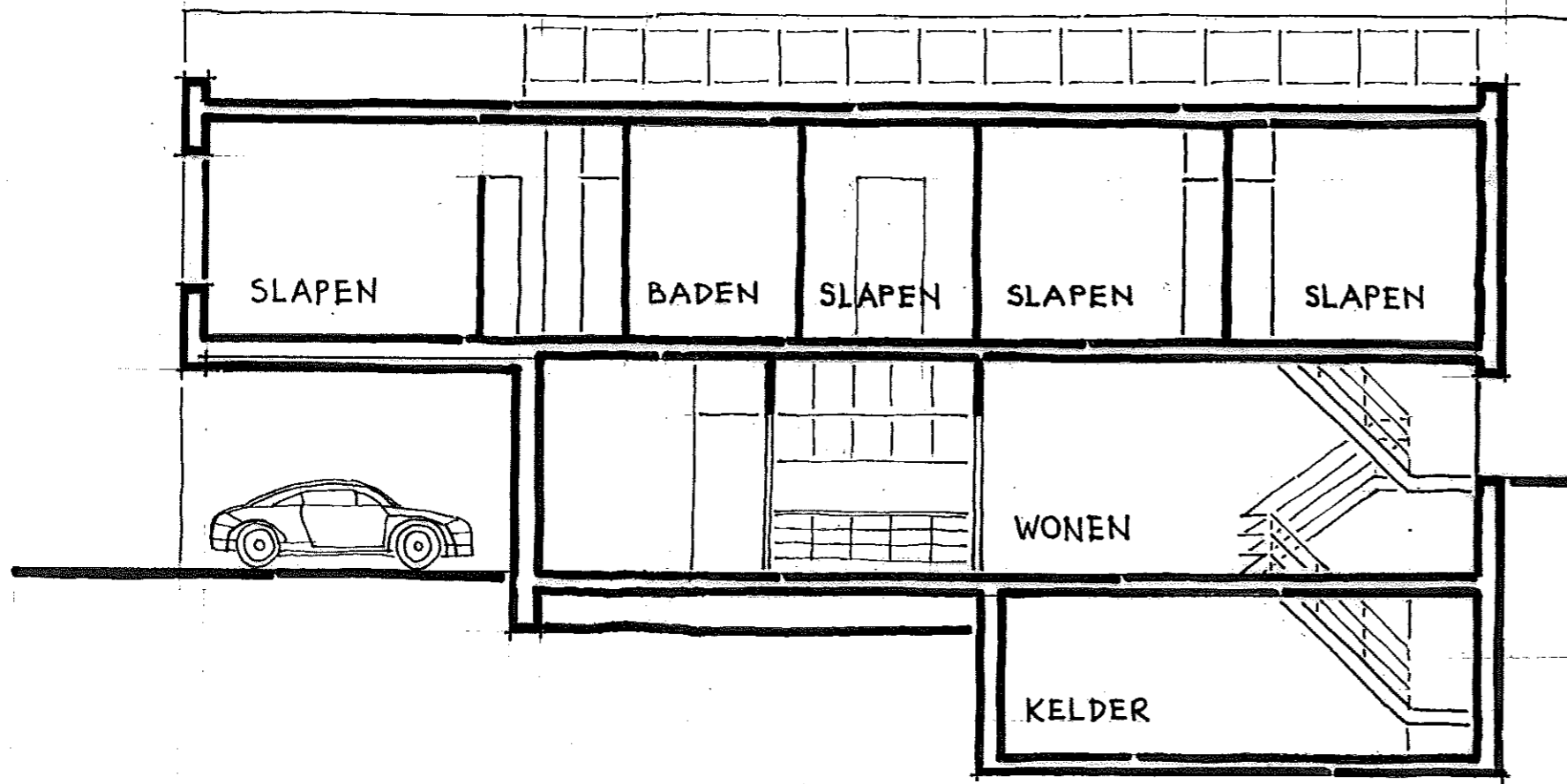
LANGSDOORSNEDE
